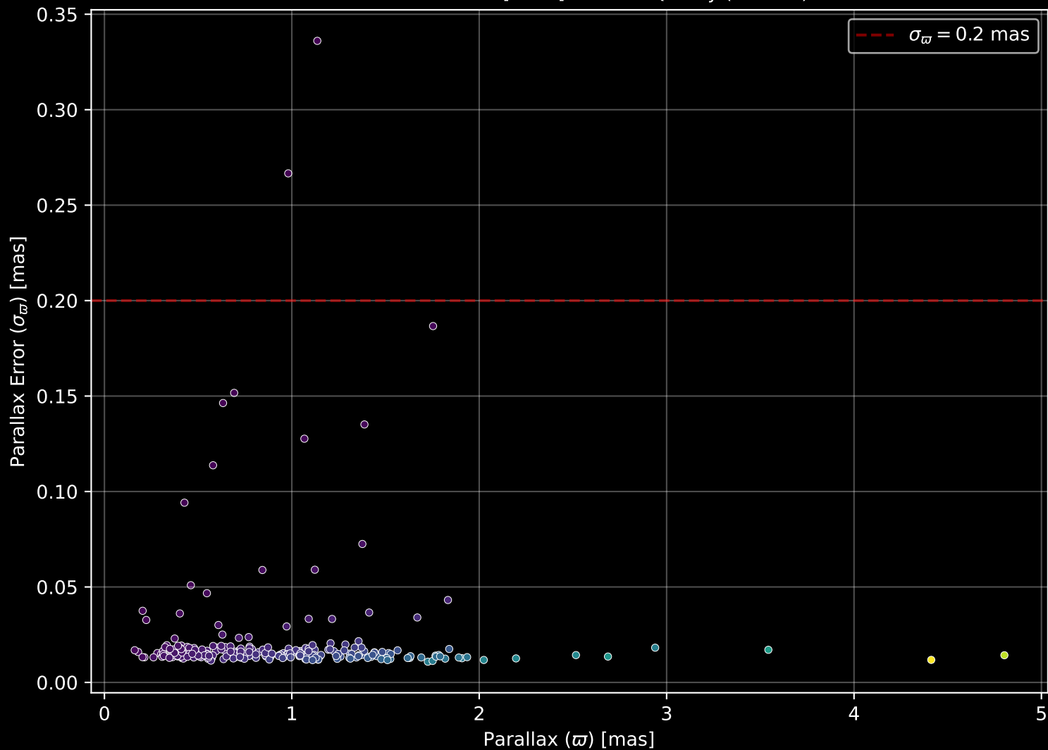
GALAH DR4 Field: [8824] Parallax Quality (n= 246)
