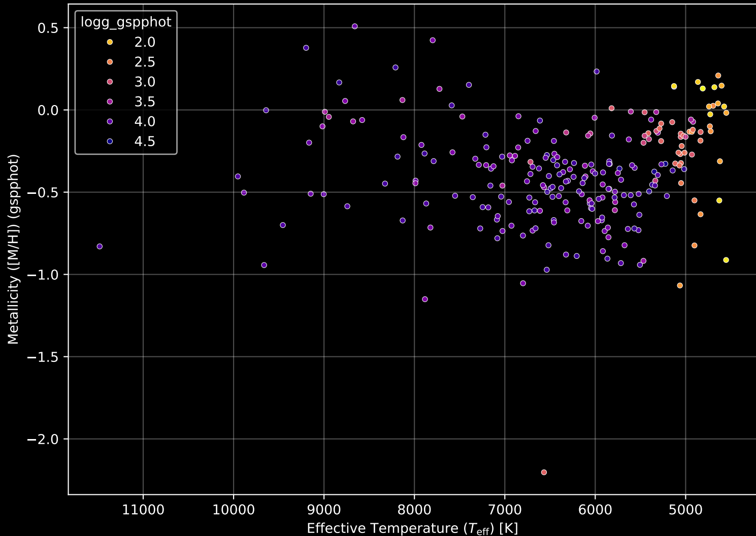
GALAH DR4 Field: [8824] Stellar Population Parameters (n= 246)
