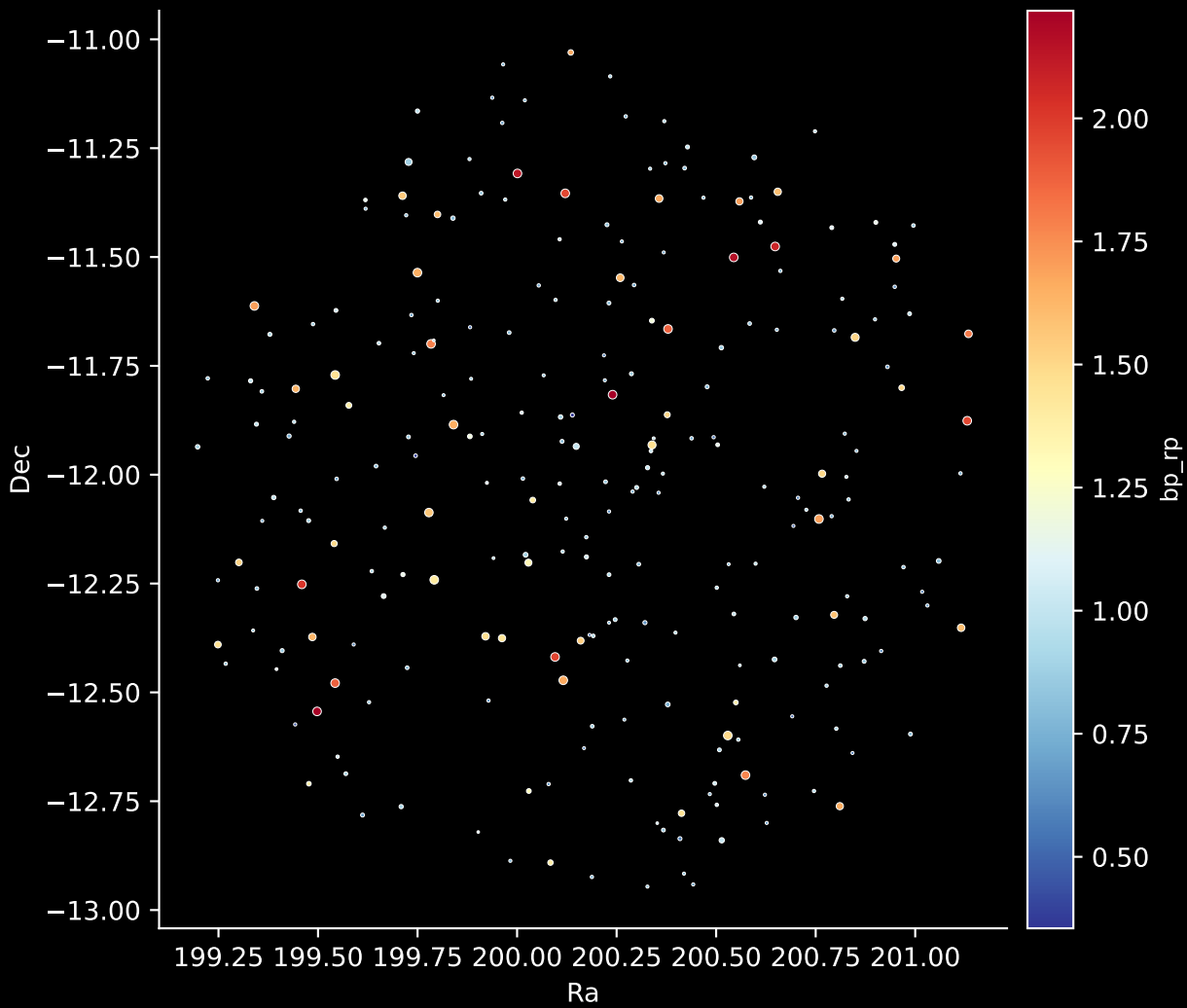
GALAH DR4 Field: [8824] Stars: 246
