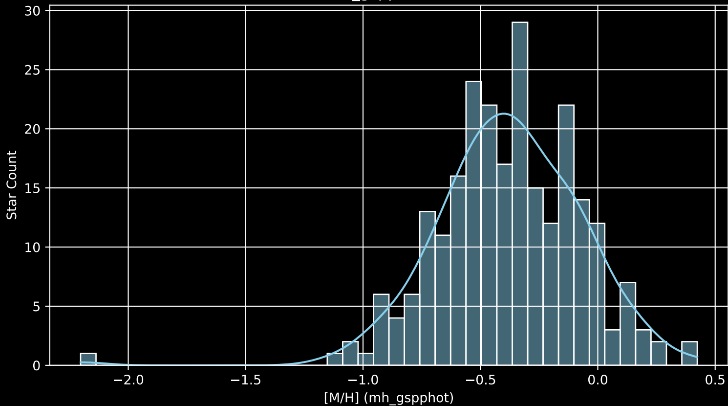
GALAH DR4 Field: [8824] [M/H] (mh_gspphot) (n= 245)
